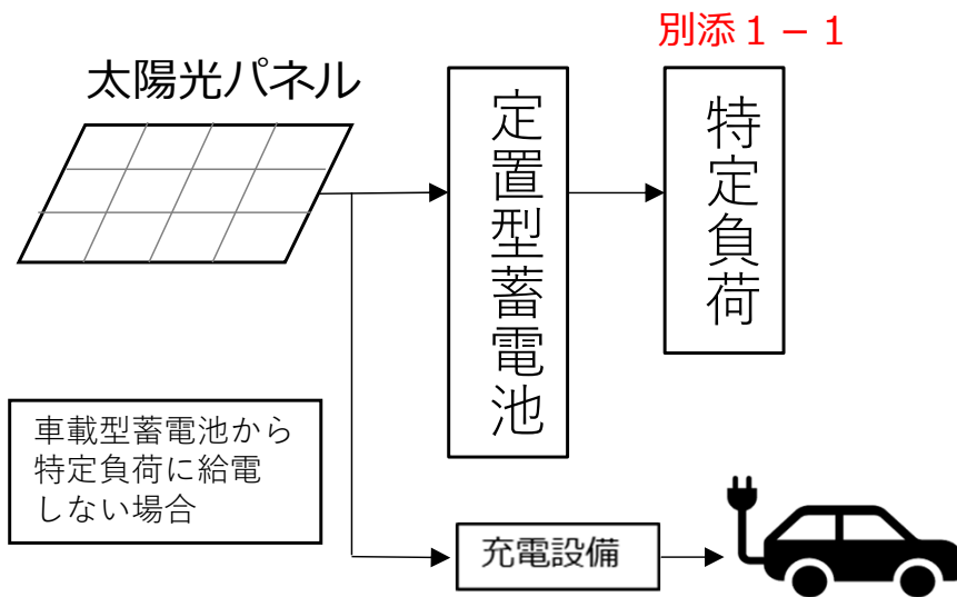
③-1 (太陽光発電設備と定置型蓄電池+車載型蓄電池)
